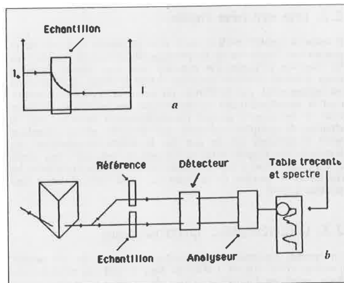
Figure 1. Schéma de principe de la spectroscopie électronique.
