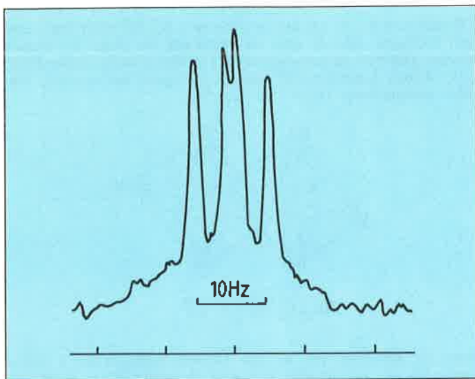
Figure 13. Spectre ^1\text{H} RMN à 400 MHz de 43.
