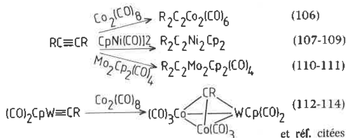
Schéma 14. Les relations isolobales sont satisfaites dans ce schéma.
