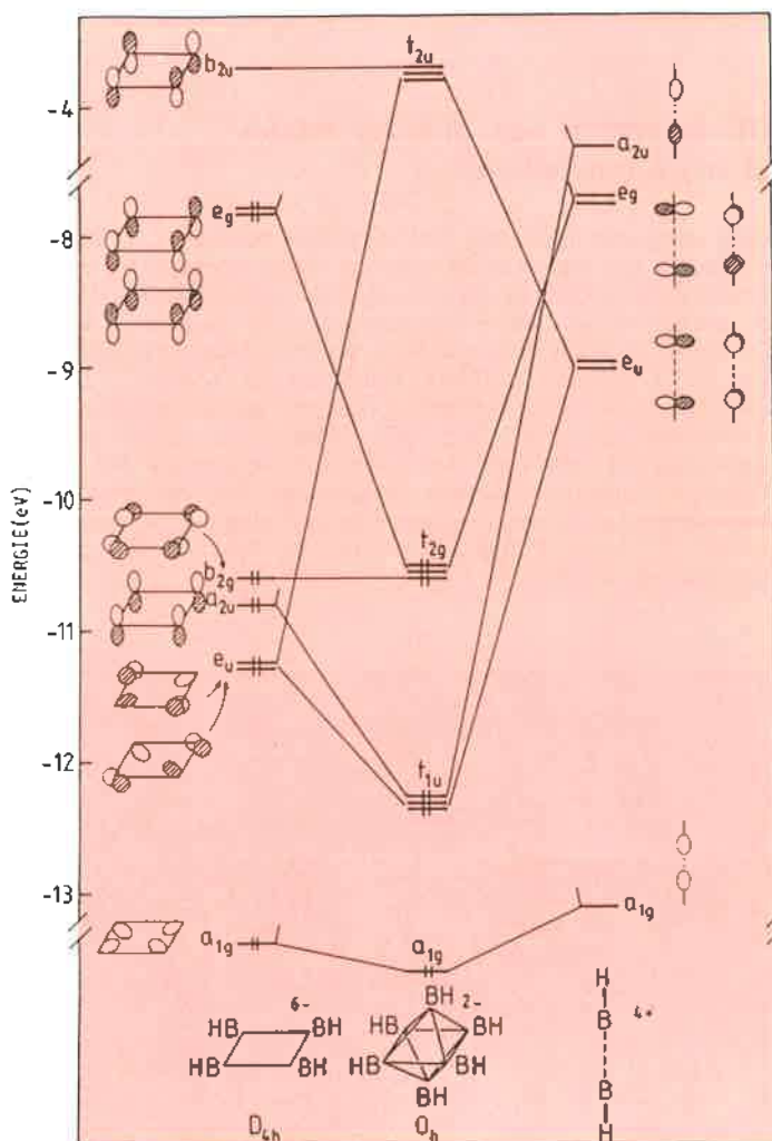
Figure 6. Diagramme d'interaction orbitaire pour B_6H_6^{2-} .
