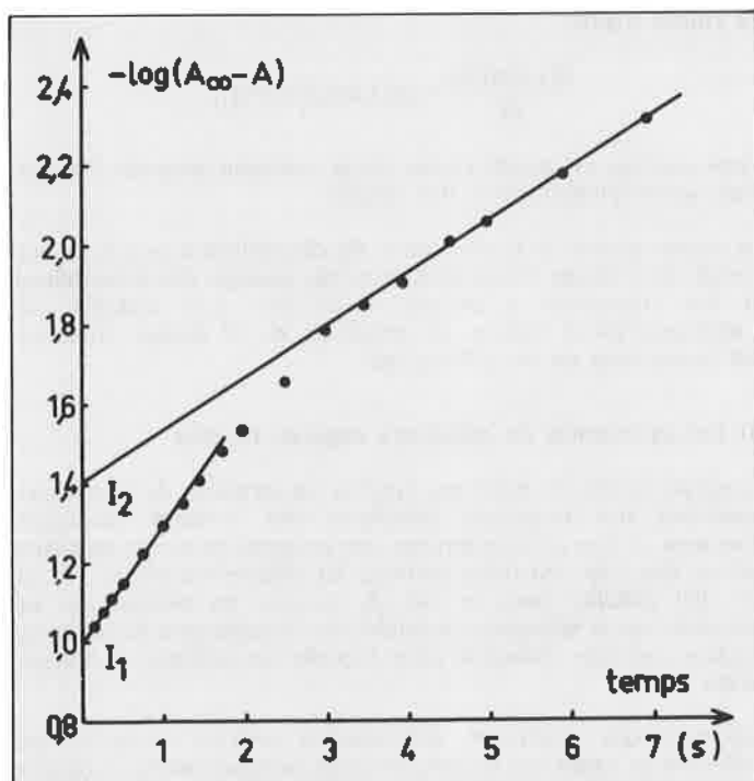
Figure 1. Extrapolation logarithmique pour le dosage par cinétique différentielle du calcium et du magnésium déplacés de leurs complexes CaCDTA et MgCDTA par le plomb (II), d'après (10).
