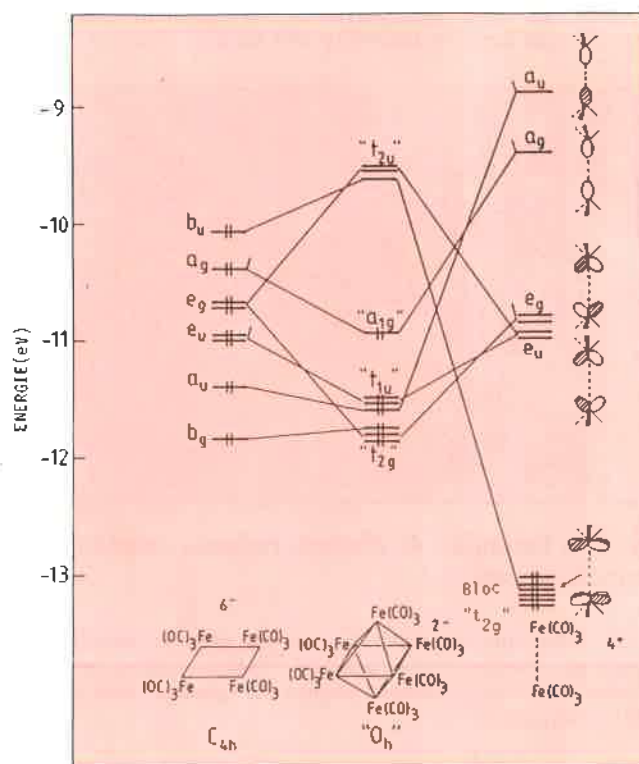
Figure 8. Diagramme d'interaction orbitale pour le cluster pseudo-octaédrique Fe(CO)_7^{2-} . Le label des niveaux moléculaires du cluster M_6 a été gardé dans le groupe de symétrie O_h .
