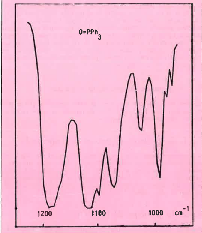
Spectre 2. Spectres infrarouge des complexes \text{CpThCl}_3(\text{OPPh}_3)_2 et \text{OPPh}_3 , entre 1250 et 950 \text{cm}^{-1} .
