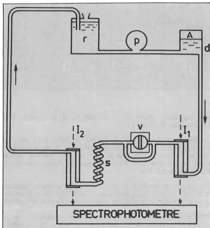
Figure 2. Dispositif expérimental. Circuit à circulation continue et fermée.
