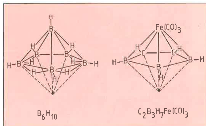
Figure 7. Le métallo-carborane C_2B_3H_7Fe(CO)_3 (14) et son analogue borane.
