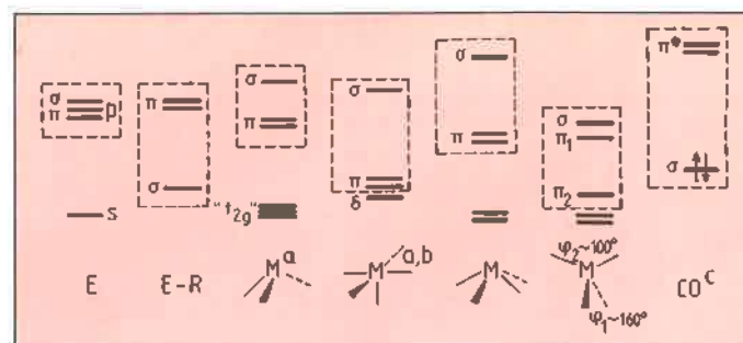
Figure 9. Quelques entités ayant un jeu similaire d'orbitales frontières. (E: élément du groupe principal, M: métal de transition). a) La structure électronique de ML_3 ou ML_5 se dérive aisément de celle d'un complexe octaédrique ML_6 (voir réf. 4). b) Si le fragment est riche en électrons, seule l'OM \sigma est considérée comme OF. c) Ou tout autre coordat isoélectronique.
