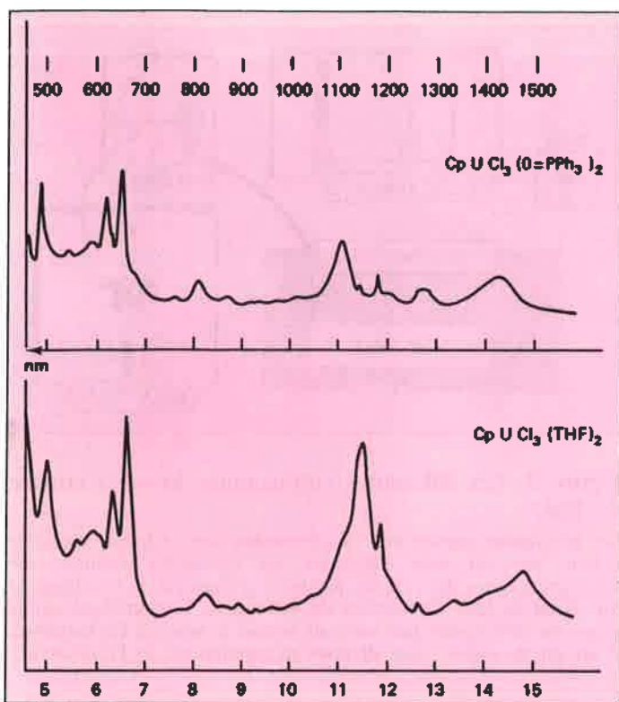
Spectre 1. Spectres électroniques (visible et proche infrarouge) des complexes \text{CpUCl}_3(\text{THF})_2 et \text{CpUCl}_3(\text{OPPh}_3)_2 .
