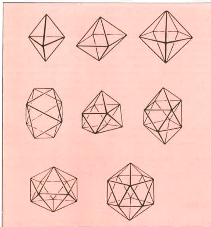
Figure 1. Quelques deltaèdres dans lesquels s'inscrivent des clusters du bore.
