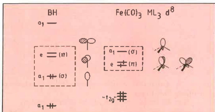
Figure 5. Analogie isobale entre B-H et Fe(CO)_3 . (L'ensemble des orbitales frontières des fragments est entouré en pointillé).
