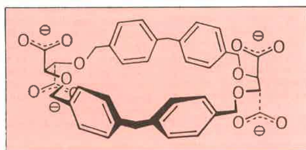
Fig. 1. Le récepteur moléculaire synthétique (ER 285).
