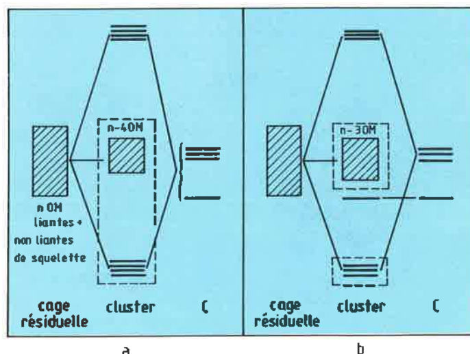
Figure 10 a) Schéma orbitalaire d'un cluster avec élément exposé ou encapsulé. b) Schéma orbitalaire d'un cluster avec un atome nu comme sommet.
