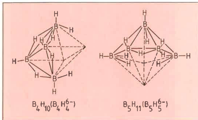
Figure 4. Exemples de clusters boranes arachno (deux sommets vacants).
