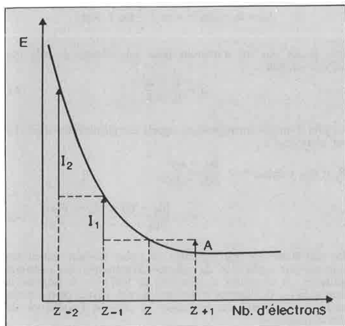
Figure 1. Variation de l'énergie totale avec le nombre d'électrons autour du noyau de numéro atomique Z.
