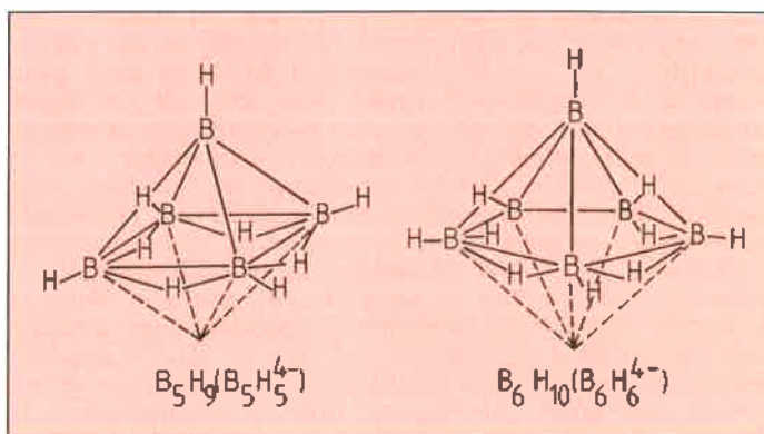
Figure 3. Exemples de clusters boranes nido (un sommet vacant).
