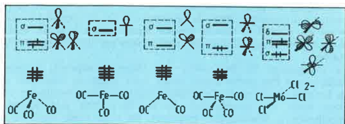
Figure 12. Comparaison des OF de fragments non coniques avec celles du fragment ML_3 conique ( C_{3v} ).
