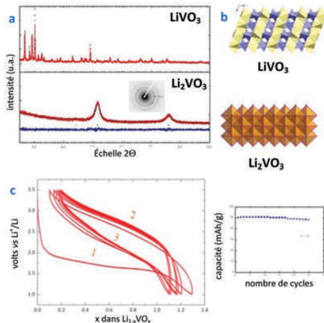
Figure 3 - (a) Diagramme de diffraction des rayons X ex situ de la phase réduite \text{Li}_2\text{VO}_3 ; (b) structure de \text{LiVO}_3 selon l'axe a; et (c) courbe potentiel/composition de \text{LiVO}_3 au régime de C/10.
