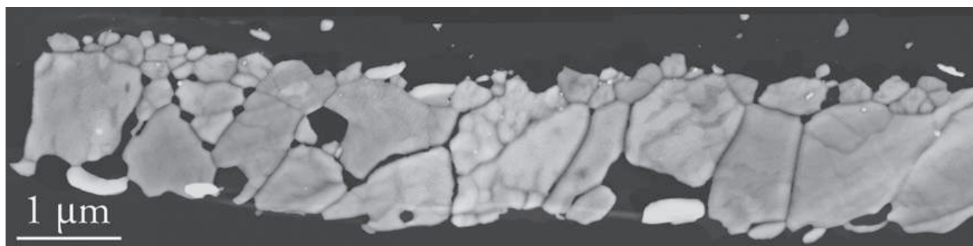
Figure 2 - Vue en coupe transversale en STEM-HAADF de la couche de sous-chlorure d'argent d'un échantillon bleu (JEOL 2100FEG, 200 kV, STEM-HAADF, taille de sonde 0,2 nm, diaphragme 50 μm ; série d'images à 50 k raboutées).
