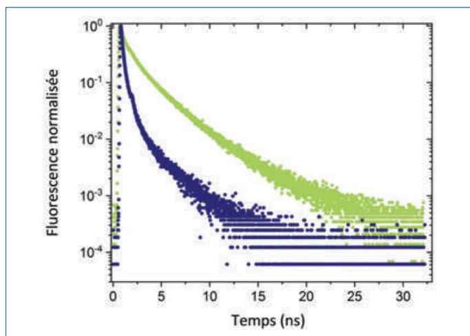
Figure 4 - Déclin de fluorescence de l'oxytréacycline libre en solution (points bleus) et confinée dans des hydroxydes doubles lamellaires (points verts).
