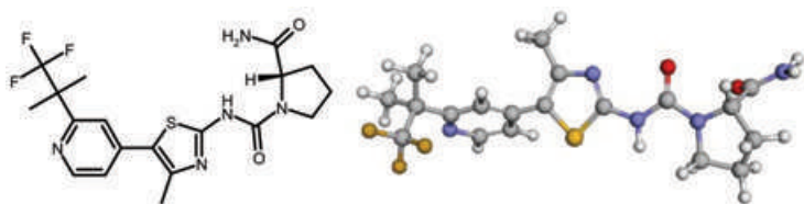
Structure de l'alpelisib (représentation 3D issue du site Drugbank, www.drugbank.ca/structures/small_molecule_drugs/DB12015 ).
