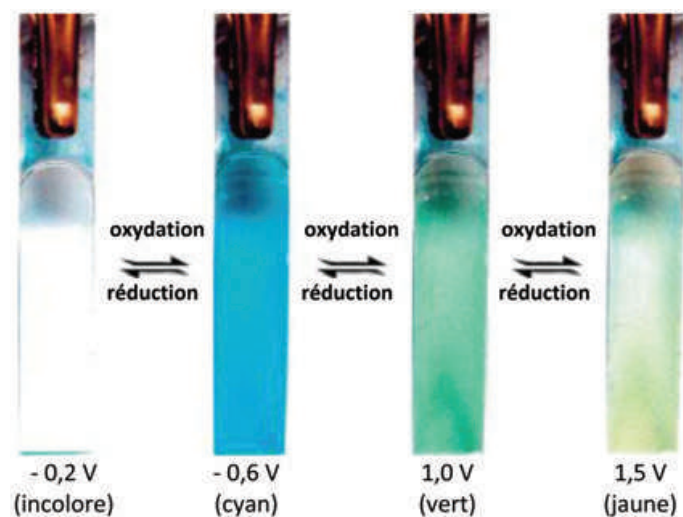
Figure 8 - Photos des films multicouches de bleu de Prusse et de polyéthylène imine à différents potentiels (image adaptée de [15]).
