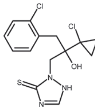
Structure du prothioconazole. N° CAS : 178928-70-6 ; nom IUPAC : (RS)-2-[2-(1-chlorocyclopropyl)-3-(2-chlorophényl)-2-hydroxypropyl]-1,2-dihydro-1,2,4-triazole-3-thione.
