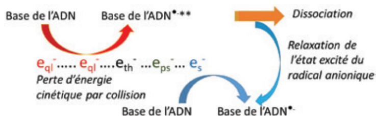
Figure 3 - Schéma représentant la réactivité de e_{qi}^- et de e_s^- avec une base de l'ADN et les deux voies possibles du déclin du radical anionique excité (base d'ADN ^{\bullet*} ): relaxation ou dissociation. Dans l'eau, la dissociation de l'anion excité n'est pas observée.
