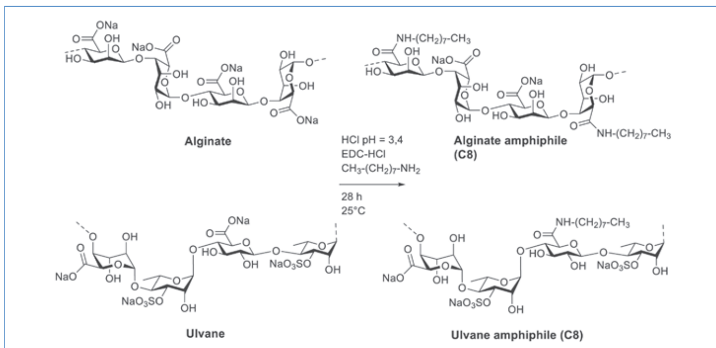
Figure 1 - Synthèse des alginate et ulvane amphiphiles dérivés de la dodécylamine par l'agent de couplage EDC-HCl. Alginate amphiphile : Rdt = 41 % ; masse molaire = 233 600 g mol -1 . Ulvane amphiphile : Rdt = 43 % ; masse molaire = 706 100 g mol -1 .
