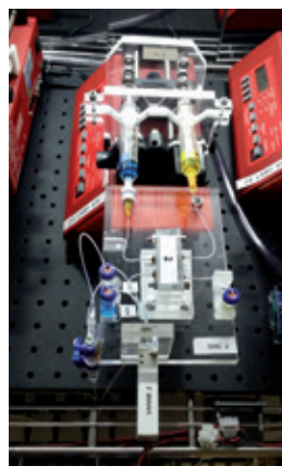
Banc instrumenté de microfluidique, actuellement opérationnel à Singapour au laboratoire CEA/NTU SCARCE, permettant de réduire à 1 mL une expérience d'extraction sélective de métaux. © CEA/ICSM.
