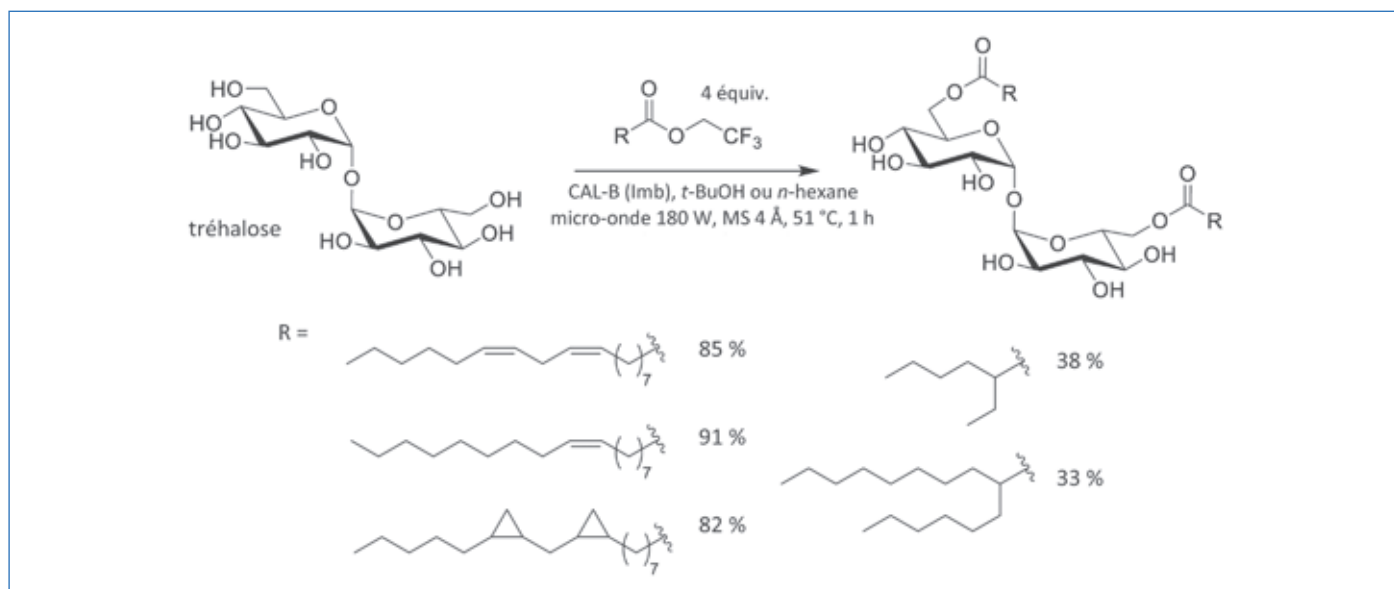
Figure 6 - Préparation des diacylthréhaloses.
