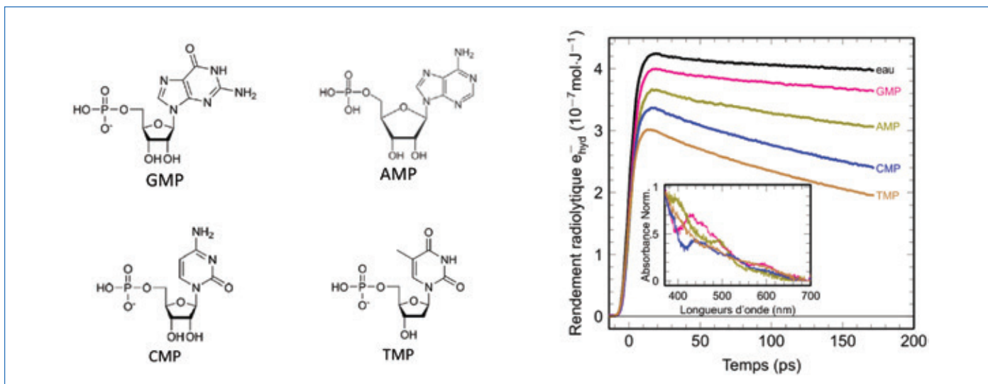
Figure 2 - Rendement radiolytique de e_{aq}^- en fonction du temps en présence de nucléotides 250 mM (GMP, AMP, CMP et TMP) dans l'eau. En encadré : les spectres d'absorption des radicaux ( GMP^{\bullet-} , AMP^{\bullet-} , CMP^{\bullet-} et TMP^{\bullet-} ) observés à 5 ps sont obtenus par soustraction appropriée du spectre d'absorption de e_{aq}^- du spectre total enregistré expérimentalement, en utilisant une analyse globale des données [18]. Adapté avec permission de [18], © 2017 American Association for the Advancement of Science.
