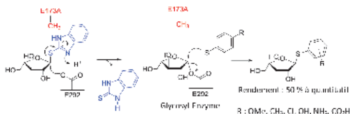
Figure 9 - Réaction de thioligation catalysée par le mutant CtAra51 E173A.
