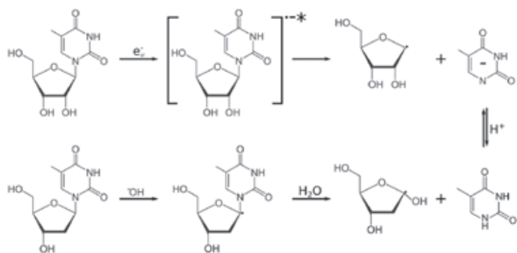
Figure 6 - Réactions entre e_{qi}^- et rT et entre le radical \cdot\text{OH} et le thymidine.
