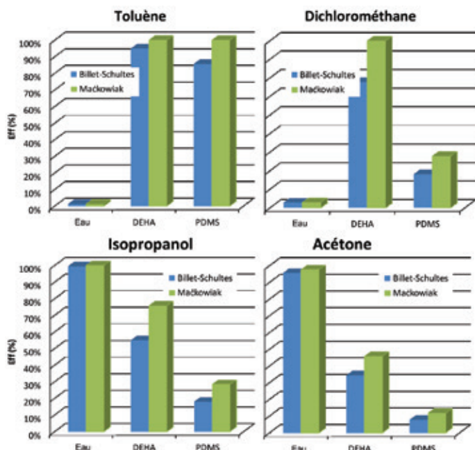
Figure 3 - Efficacité d'élimination modélisée en utilisant les théories de Billet-Schultes et de Mačkowiak.
