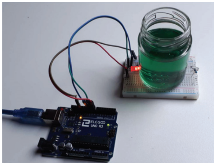
Figure 1 - Colorimètre LED-Arduino-photodiode trois couleurs utilisé pour l'étude de la cinétique de disparition des colorants dans un sirop de menthe.
