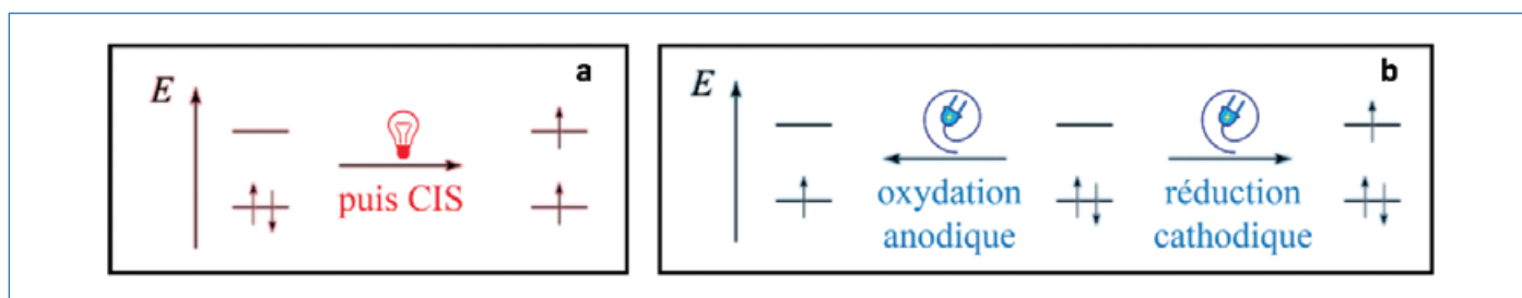
Figure 2 - Diagramme orbitalaire simplifié dans le cadre d'une excitation photochimique (a) et d'une oxydation/réduction électrochimique (b). CIS : conversion intersystème.
