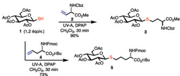
Figure 3 - Synthèse de S-glycosyl-aminoacides par couplage thiol-ène.
