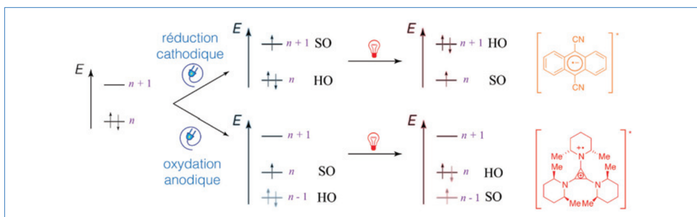
Figure 12 - Inversion des orbitales HO-SO en électrophotocatalyse pour les deux catalyseurs présentés.
