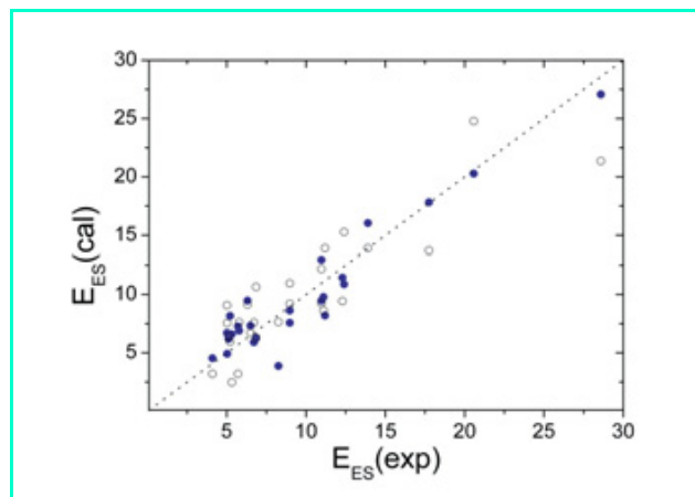
Figure 4 - Sensibilités électriques (en J) calculées selon l'équation (EQ4) (●) et selon le modèle de Keshavarz [25] (○) en fonction des valeurs expérimentales.
