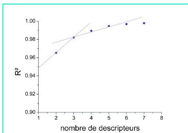
Figure 2 - Définition du nombre optimal de descripteurs dans le modèle.
