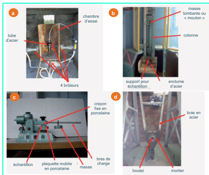
Figure 1 - Exemples d'appareillages permettant l'évaluation des substances explosibles selon le Manuel d'épreuves et de critères [6] et le règlement des méthodes d'essai européen [4] : épreuve a) de Koenen, b) de sensibilité à l'impact, c) de sensibilité au frottement, d) du mortier balistique.
