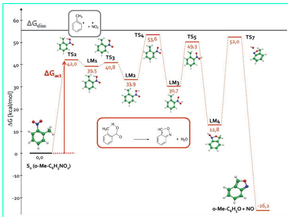
Figure 5 - Mécanismes de décomposition de l'ortho-nitrotoluène calculés à l'aide de la DFT [27].
