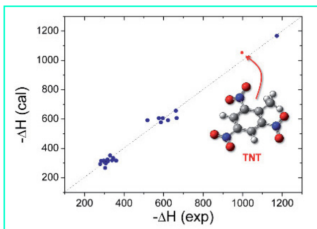
Figure 3 - Chaleurs de décomposition calculées à partir du modèle (EQ2) en fonction des valeurs expérimentales.
