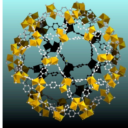
Hybrid mesoporous solid : MIL-101
