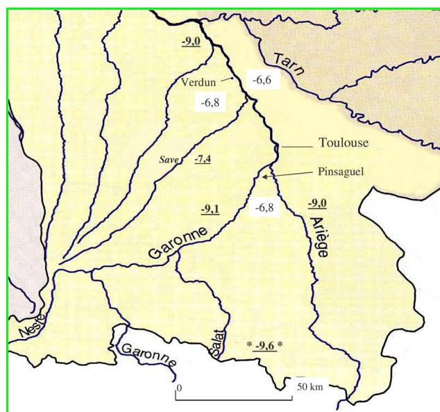
Figure 1 - Valeurs isotopiques ^{18}\text{O} des eaux autour de Toulouse (en fond blanc : eau de nappe).
